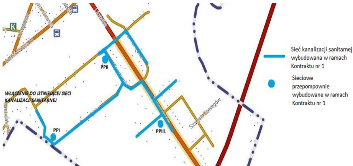
Sieć kanalizacji sanitarnej i rozmieszczenie przepompowni wybudowanych w ramach Kontraktu nr 1.
