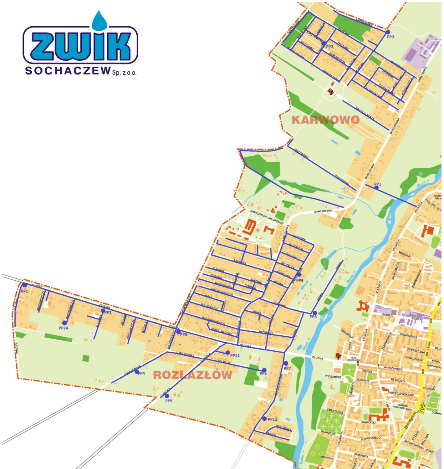
Trasa sieci kanalizacji sanitarnej i rozmieszczenie pompowni wybudowanych w ramach Kontraktu nr 2.
