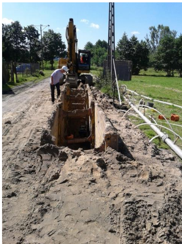
Prace przy budowie kanalizacji sanitarnej w ul. Pasaż Duplickiego
