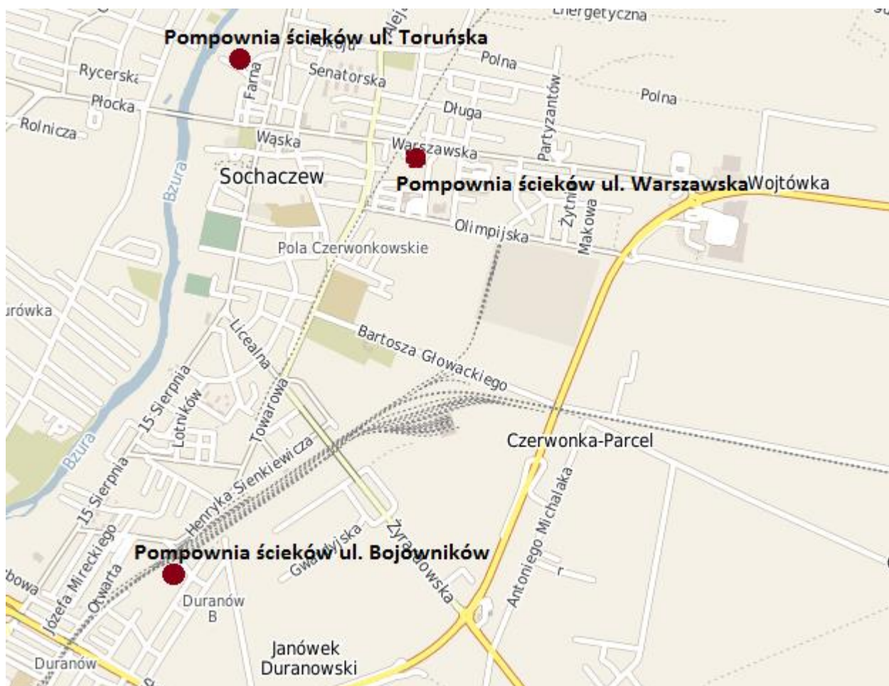
Rys. nr 3. Lokalizacja pompowni ścieków dla których prowadzono roboty w ramach Kontraktu nr 6.
