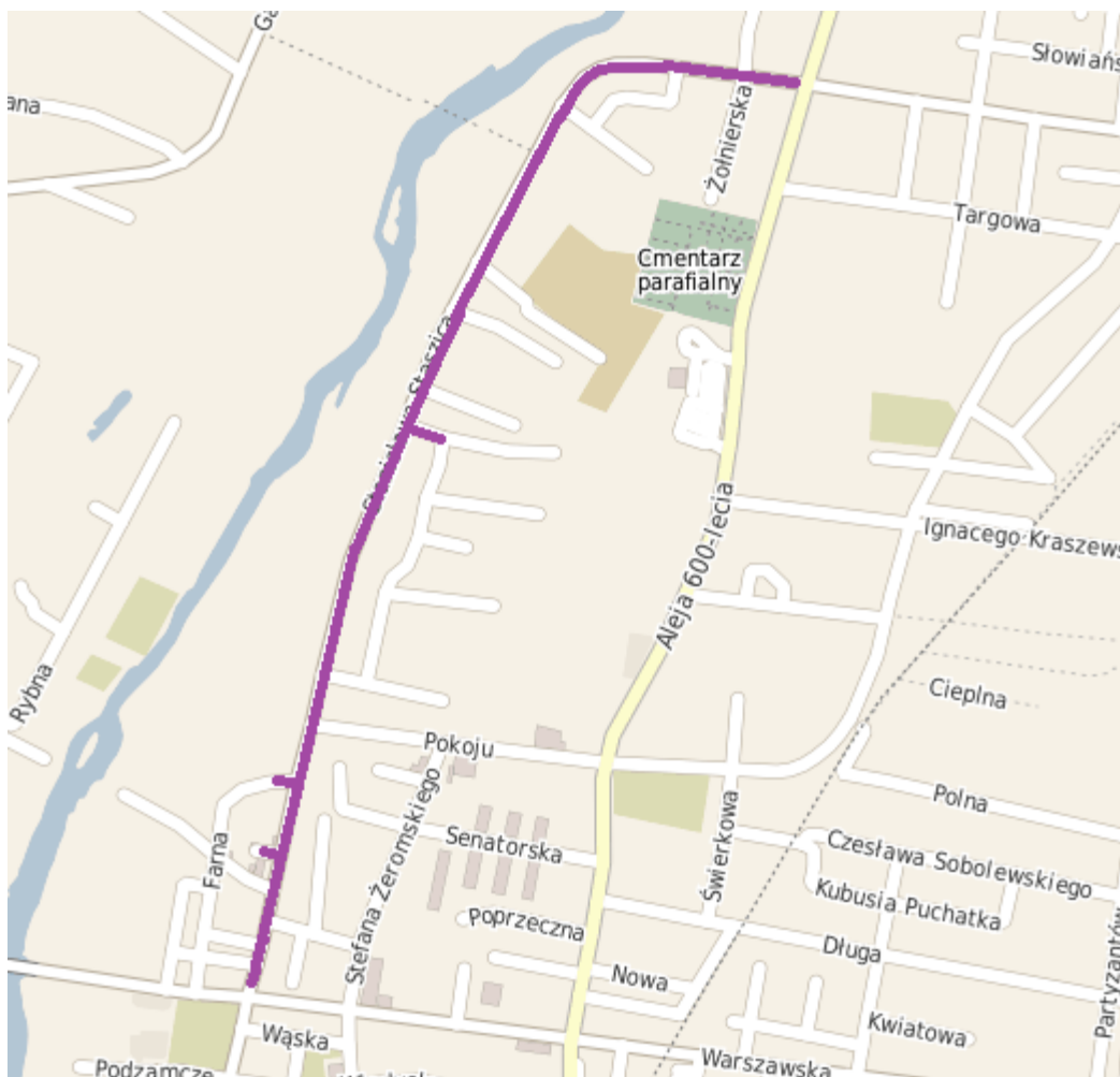
Rys. nr 2. Lokalizacja budowy i przebudowy sieci wodociągowej rozdzielczej wraz z przyłączami oraz renowacji kanalizacji sanitarnej wraz z budową przyłączy przeprowadzonych w ramach Kontraktu nr 5.
