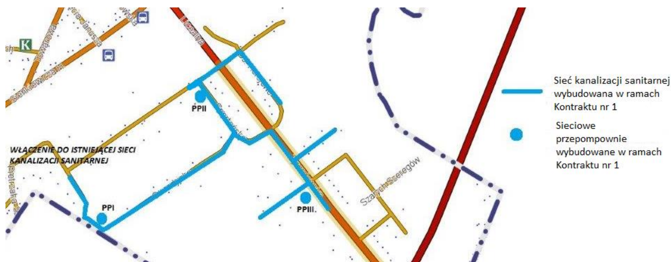
Rys. nr 1. Sieć kanalizacji sanitarnej i rozmieszczenie przepompowni wybudowanych w ramach Kontraktu nr 1.
